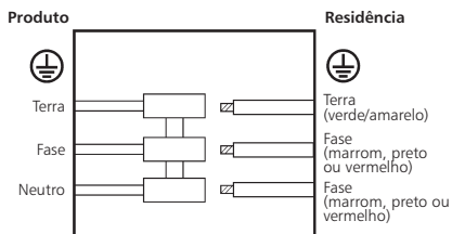
LIGAÇÃO FASE-FASE (220 V)
