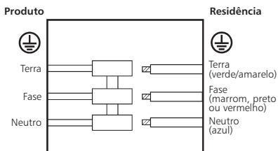
LIGAÇÃO FASE-NEUTRO (220 V)
